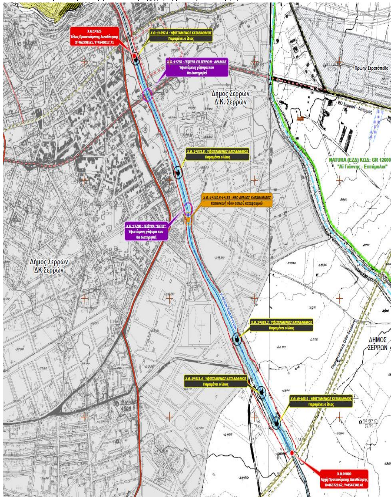
Εικόνα 1: Προτεινόμενα έργα διευθέτησης χειμάρρου Αγίων Αναργύρων
