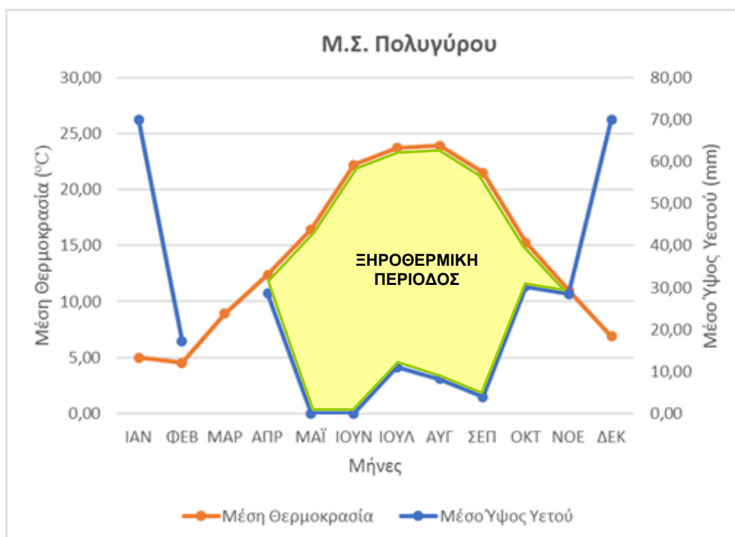
Σχήμα 6-7: Ομβροθερμικό διάγραμμα Gaussen – Bagnouls για τον Μ.Σ. Πολυγύρου
