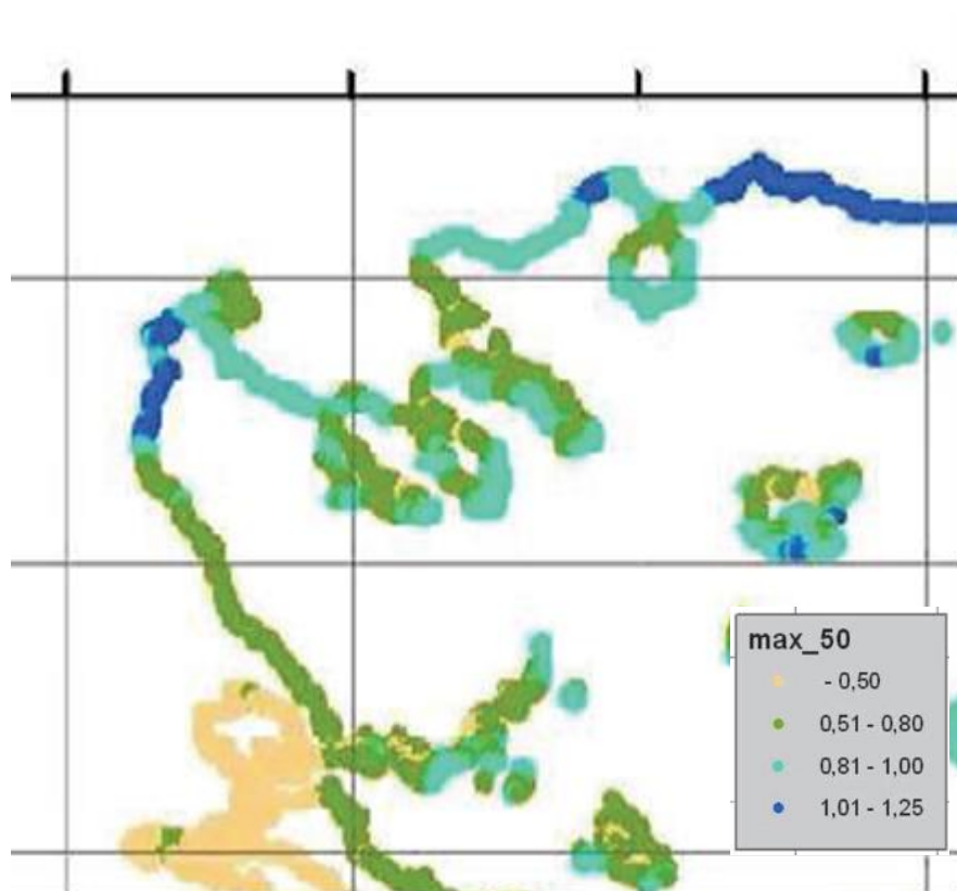
Εικόνα 6-40: Συνολική μέγιστη ανύψωση Μέσης Στάθμης Θάλασσας (ΜΣΘ) στην ακτογραμμή της περιοχής μελέτης, από όλες τις διευθύνσεις, για T=50 έτη.
