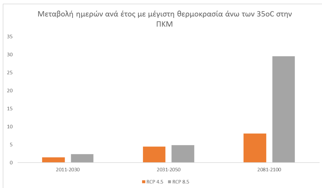
Σχήμα 4-6: Μεταβολή του αριθμού ημερών με T_{max} > 35^{\circ}\text{C} , για κάθε σενάριο παγκόσμιας εξέλιξης συγκεντρώσεων ΑΦΘ και χρονική περίοδο, σε σχέση με την περίοδο αναφοράς
