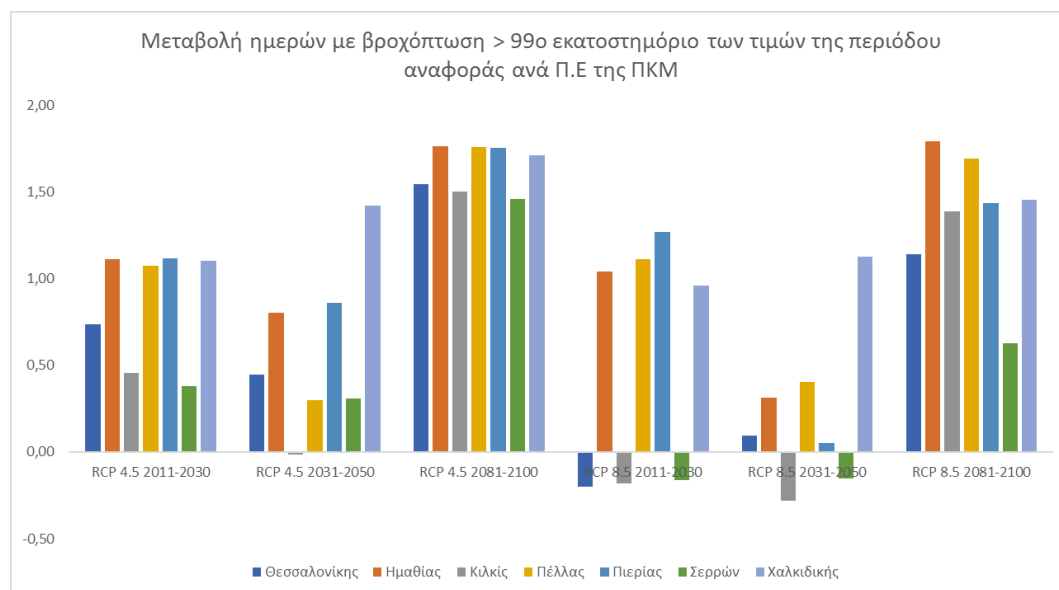
Σχήμα 4-8: Μεταβολή του αριθμού ημερών με βροχόπτωση > 99ο εκατοστημόριο των τιμών της περιόδου αναφοράς (ακραία βροχόπτωση), για κάθε σενάριο παγκόσμιας εξέλιξης συγκεντρώσεων ΑΦΘ και χρονική περίοδο
