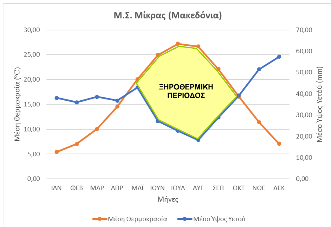
Σχήμα 6-6: Ομβροθερμικό διάγραμμα Gaussen – Bagnouls για τον Μ.Σ. Μίκρας (Μακεδονία)
