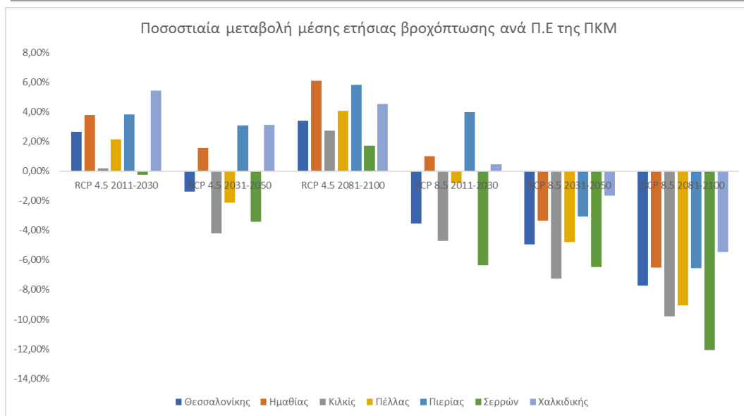
Σχήμα 4-5: Ποσοστιαία μεταβολή της μέσης ετήσιας βροχόπτωσης (%) σε επίπεδο Περιφερειακής Ενότητας, για κάθε σενάριο παγκόσμιας εξέλιξης συγκεντρώσεων ΑΦΘ και χρονική περίοδο, σε σχέση με την περίοδο αναφοράς
