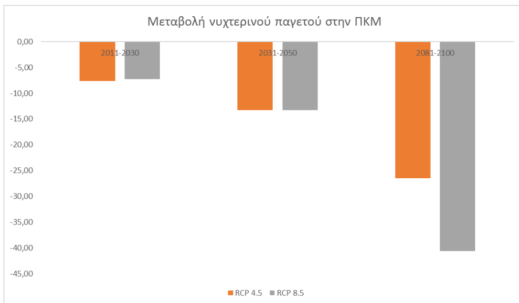
Σχήμα 4-9: Μεταβολή αριθμού ημερών με νυχτερινό παγετό (ελάχιστη θερμοκρασία < 0^{\circ}\text{C} ), για κάθε σενάριο παγκόσμιας εξέλιξης συγκεντρώσεων ΑΦΘ και χρονική περίοδο, σε σχέση με την περίοδο αναφοράς
