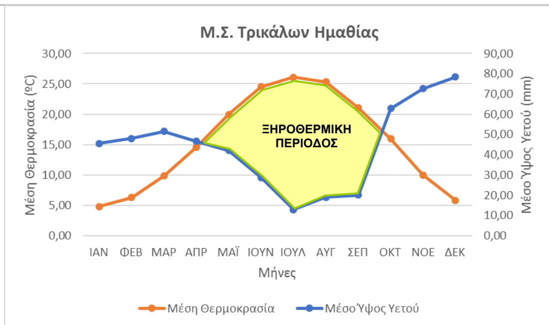
Σχήμα 6-10: Ομβροθερμικό διάγραμμα Gaussen – Bagnouls για τον Μ.Σ. Τρικάλων Ημαθίας
