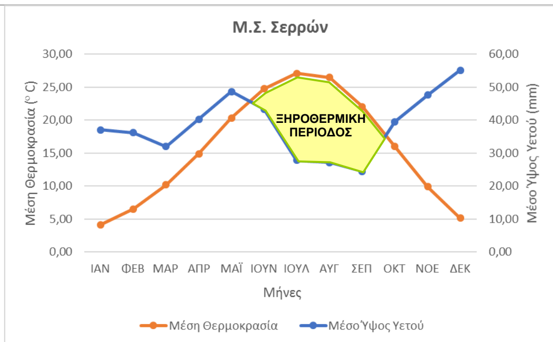
Σχήμα 6-8: Ομβροθερμικό διάγραμμα Gaussen – Bagnouls για τον Μ.Σ. Σερρών
